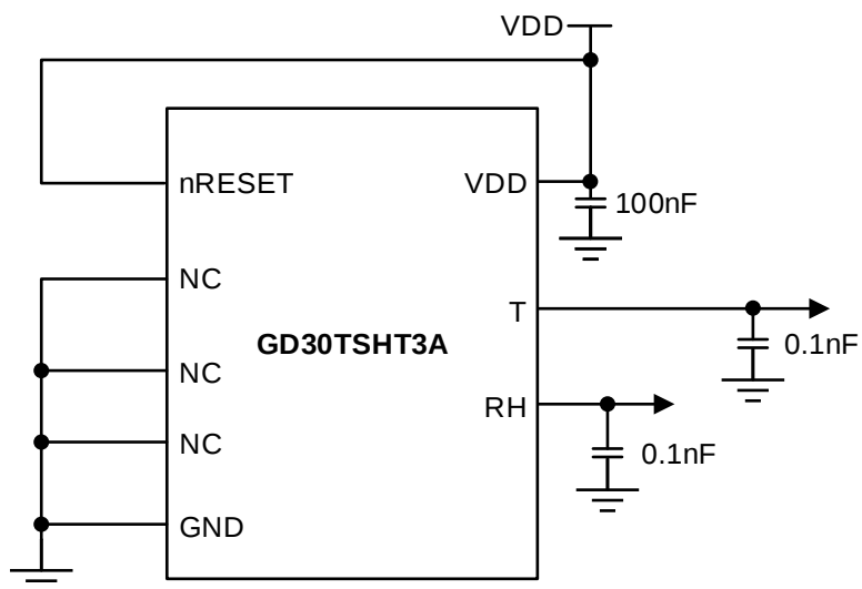
图 6. GD30TSHT3A 典型参考电路
