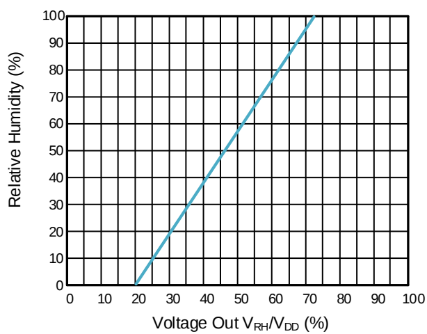
图 5. 相对湿度与输出模拟电压之间的曲线
