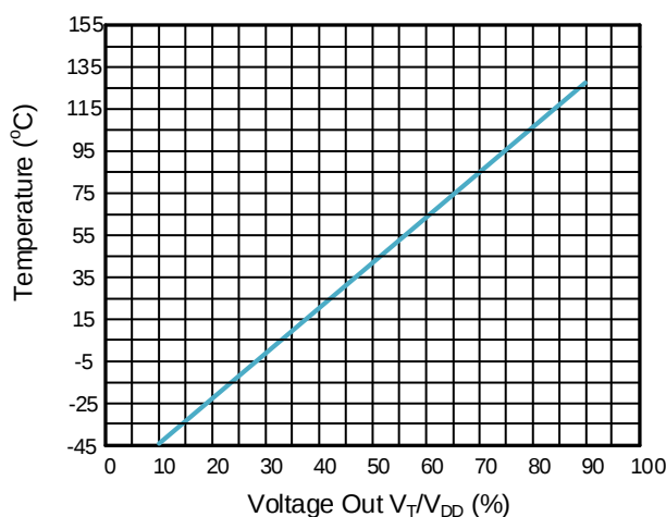
图 4. 相对温度与输出模拟电压之间的曲线
