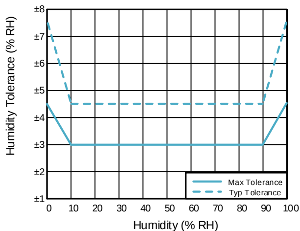
图 1. GD30TSHT3A 湿度误差
