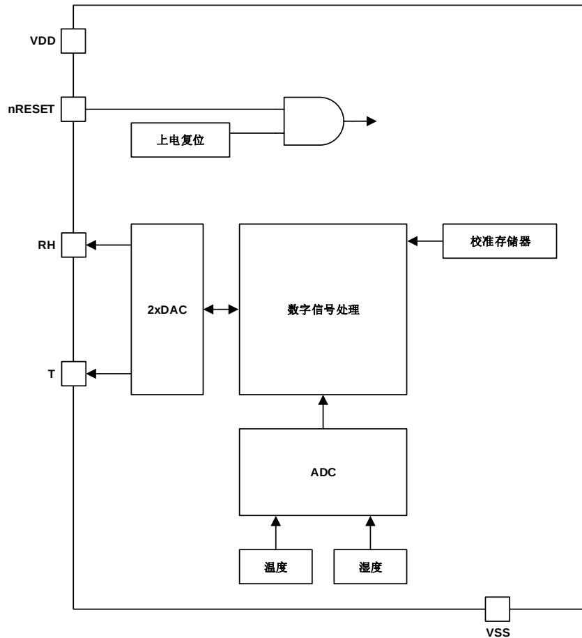
图 3. GD30TSHT3A 结构框图
