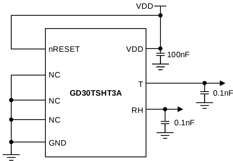
典型电路图
