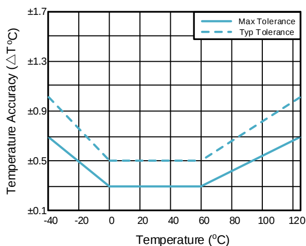
图 2. GD30TSHT3A 温度误差
