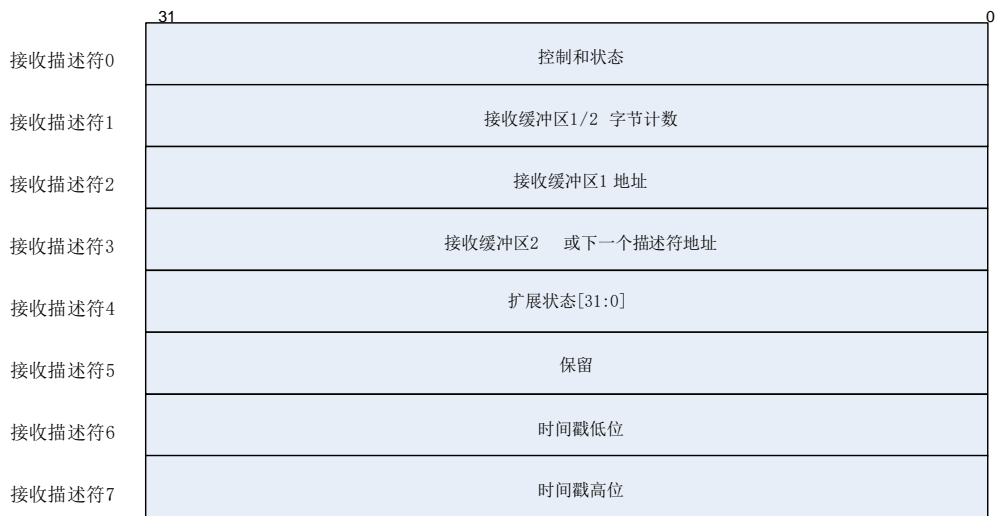
图 27-10. 增强接收描述符
