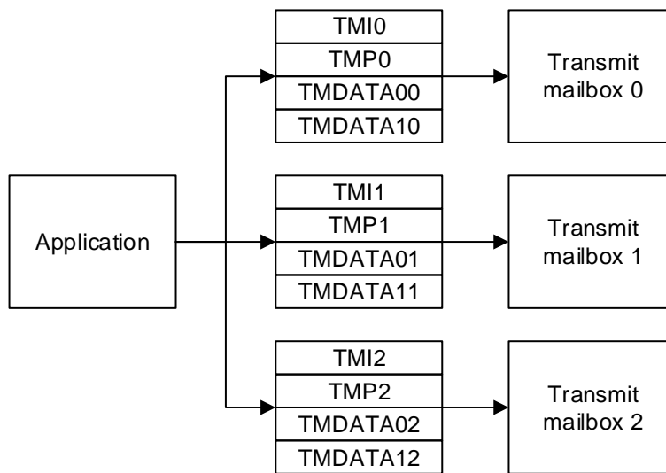
图 26-2. 发送寄存器
