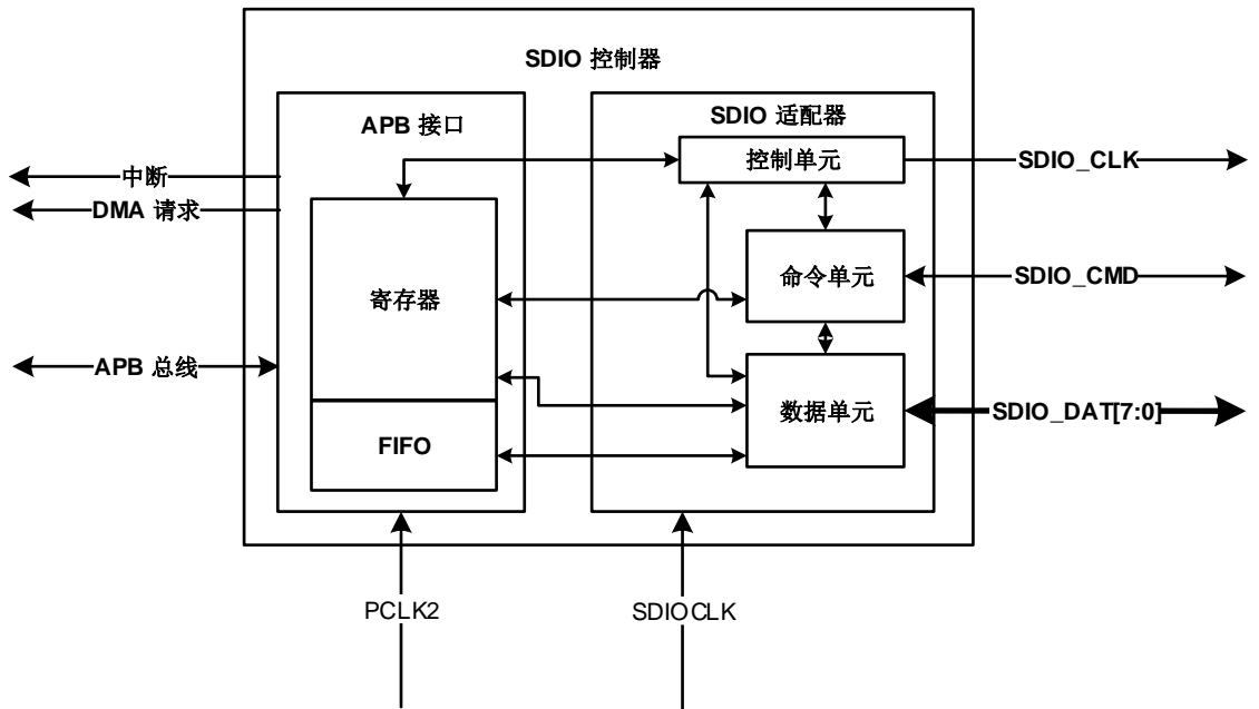
图 24-6. SDIO 框图
