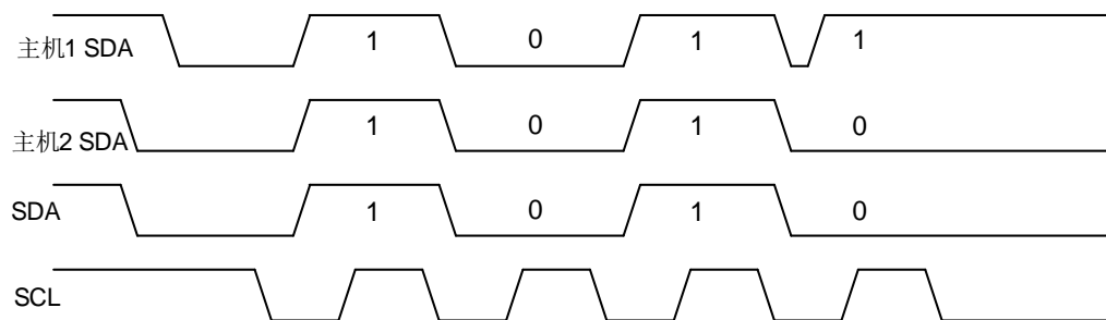
图 20-5. SDA 线仲裁
