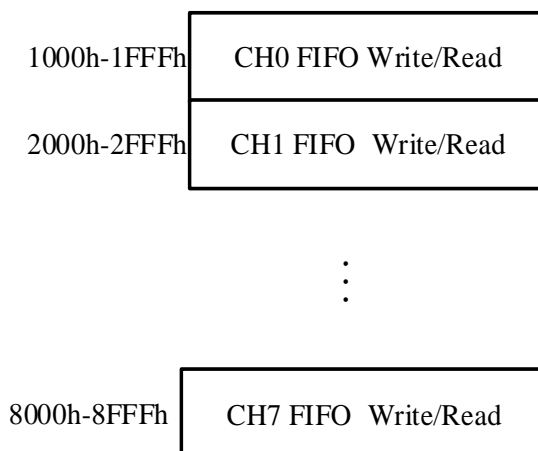
图 28-6. 主机模式 FIFO 访问寄存器映射表
