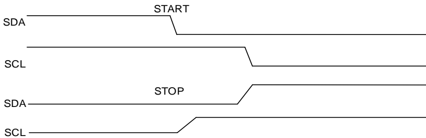
图 20-3. 起始和停止信号
