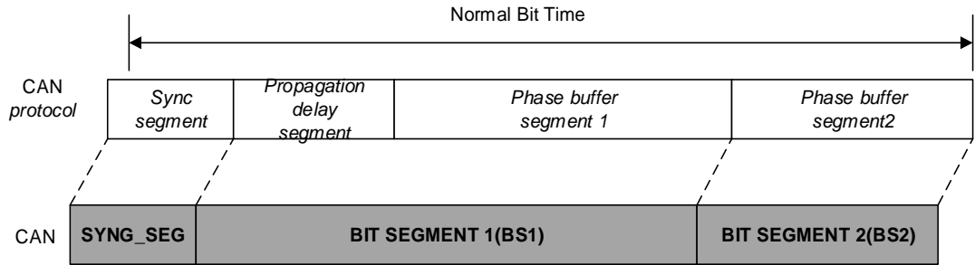
图 26-11. 位时序
