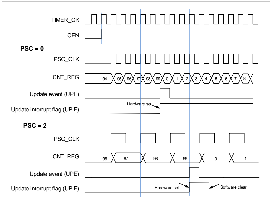
图 18-46. 向上计数时序图，PSC=0/2
