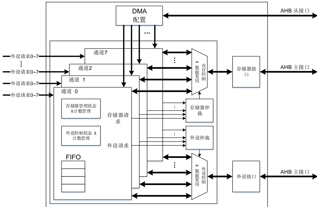
图 10-1. 系统架构
