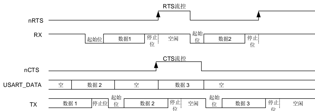
图 19-8. 硬件流控制
