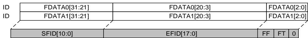
图 26-9. 32-bit 位宽列表模式过滤器
