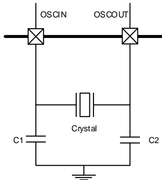
图4-3. HXTAL时钟源
