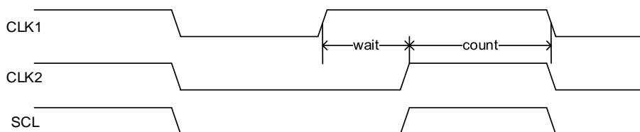
图 20-4. 时钟同步
